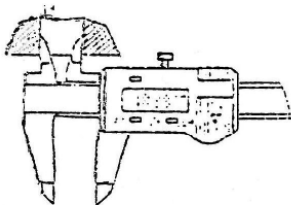
D = Misura di spallamento
